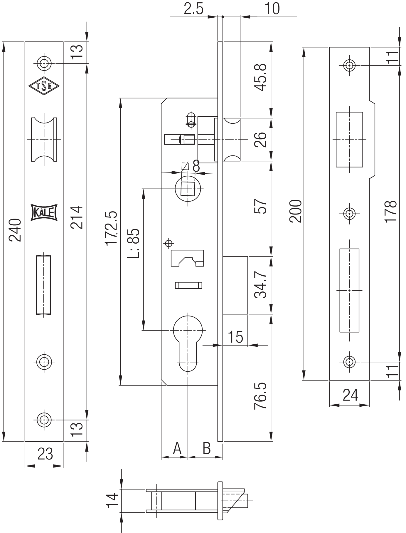
Açık Gövde Opened case
